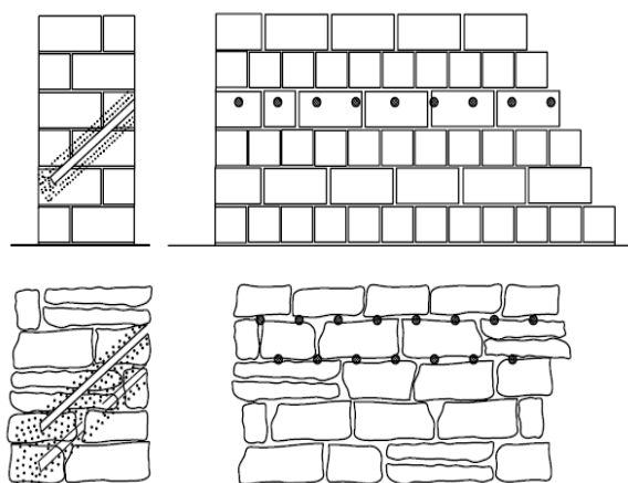
Przykład rozmieszczenia otworów - iniekcja ciśnieniowa
